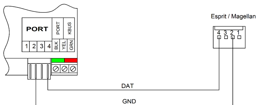
Paneļu Esprit (režīms Esprite ) vai Magellan (režīms Magellan ) pieslēgšana
