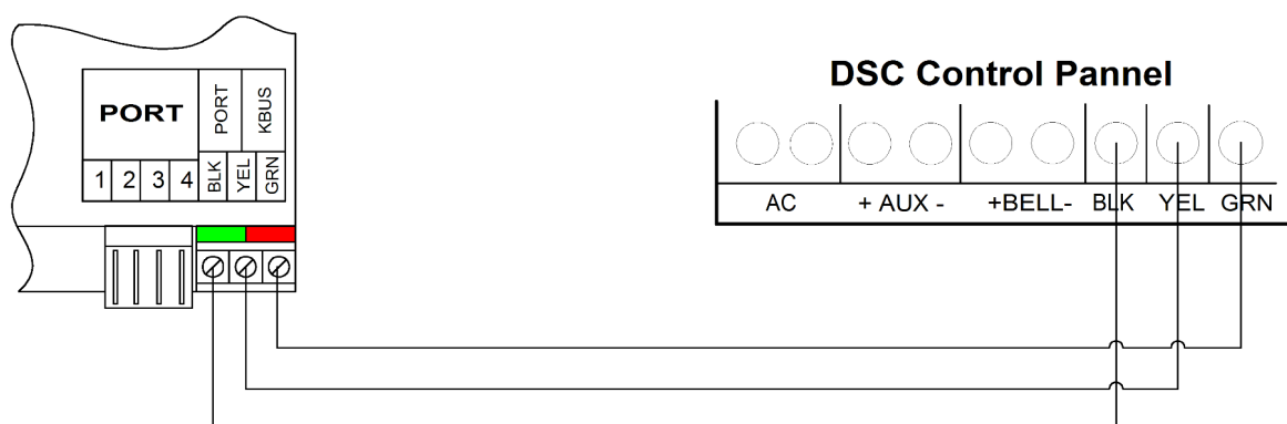
Paneļu DSC (režīms DSC ) pieslēgšana pie šinas Key-BUS
