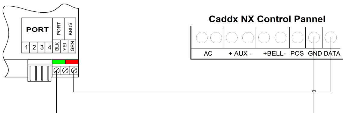
Paneļu CADDX NX (režīms NX ) pieslēgšana
