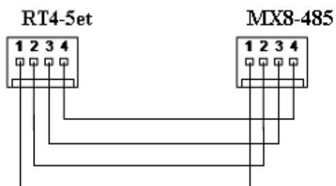
Подключение расширителя MX-8 или одного расширителя MX8-485 (режим ABUS II)
