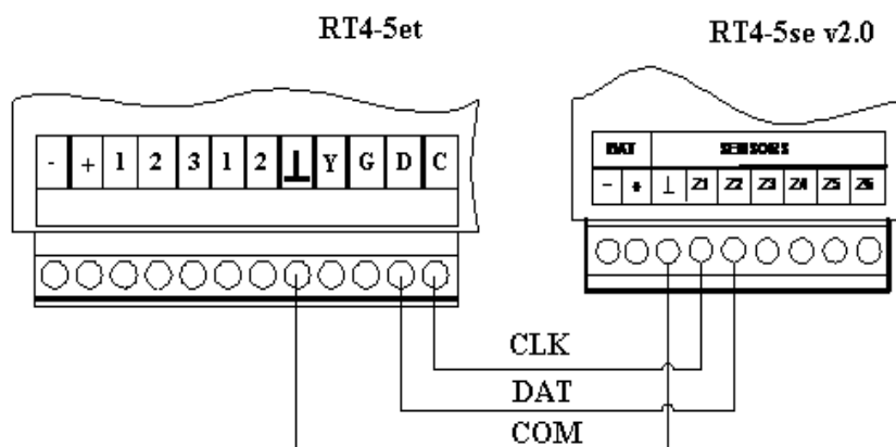
Подключение передатчика RT4-5se v.2.0
