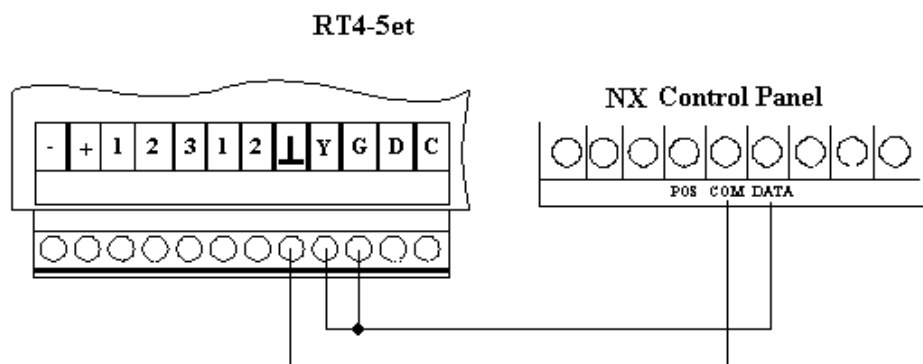
Подключение передатчика к шине панели NX (режим CADDX NX)
