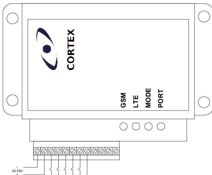
Рис.6: Подключение входов модуля.
