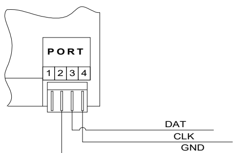
Рис.4: Подключение Serial BUS (Standard).
