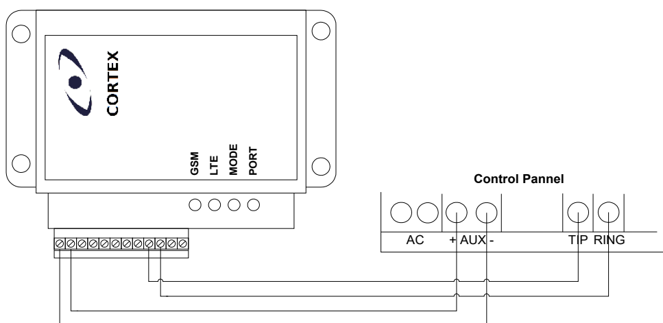
Рис.5: Подключение к PSTN коммуникатору панели.
