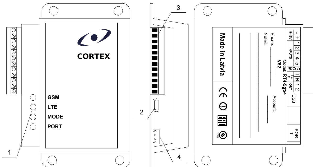
Рис. 1: Модуль RT4-5GT/4.
