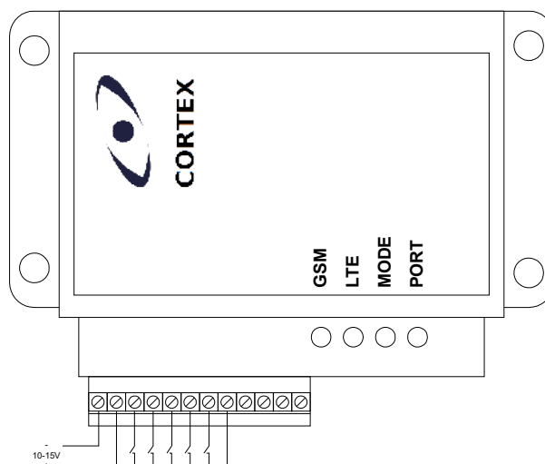
Рис. 6: Подключение входов модуля.
