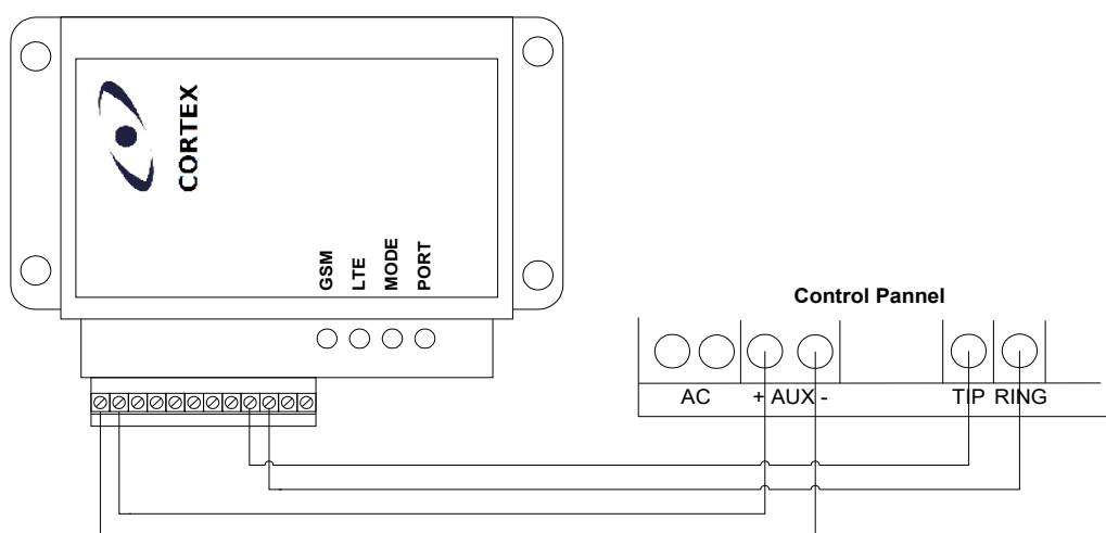
Рис. 5: Подключение к PSTN коммуникатору панели.
