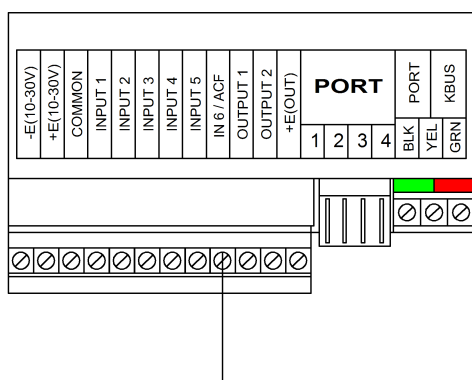
Подключение охранных шлейфов в режиме EOL
