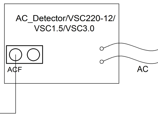
Подключение входа ACF в режиме NC/EOL
