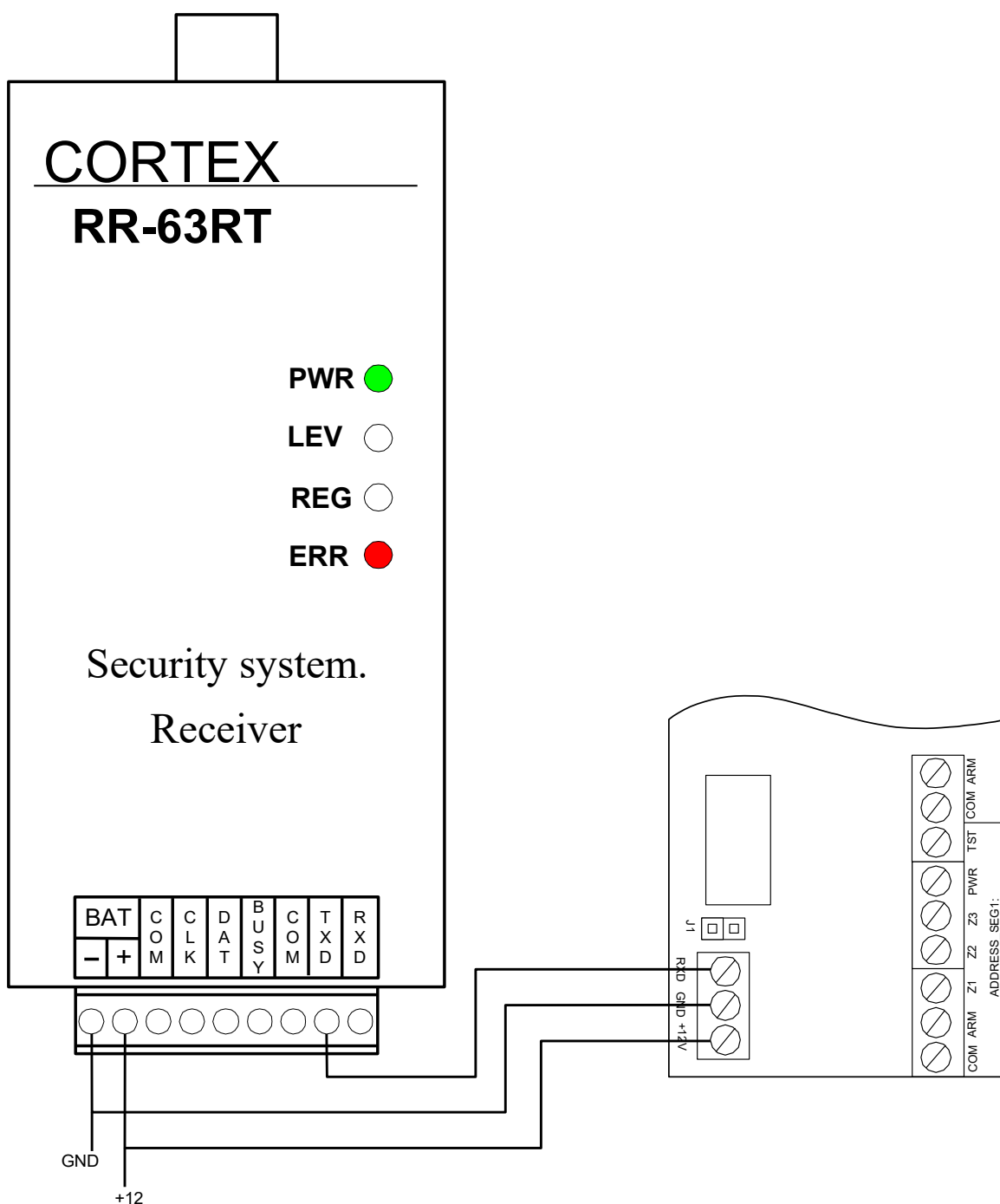
18. Zīm. PM-4 pieslēgšana raidītājam RR-63RT
