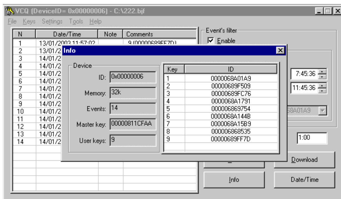
Рис. 8: Окно Info
