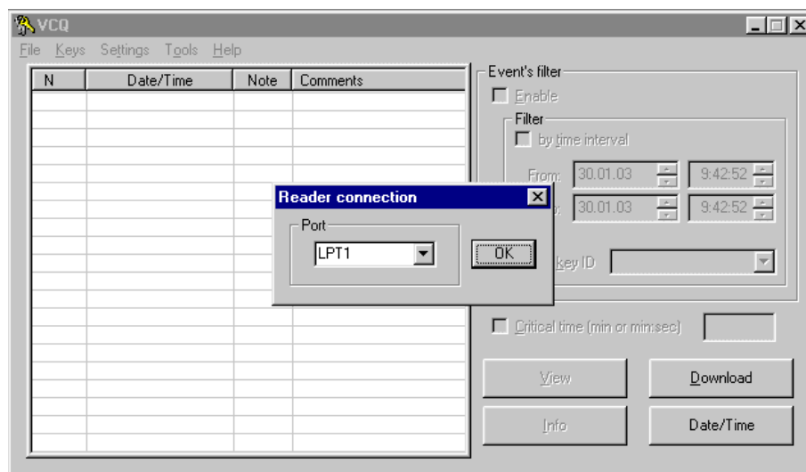
Рис. 2: Подменю Connection
